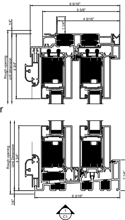
Door cut sections 1 : 4
