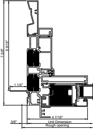
6 9/16" Jamb
