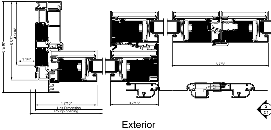
Door cut sections 1 : 4
