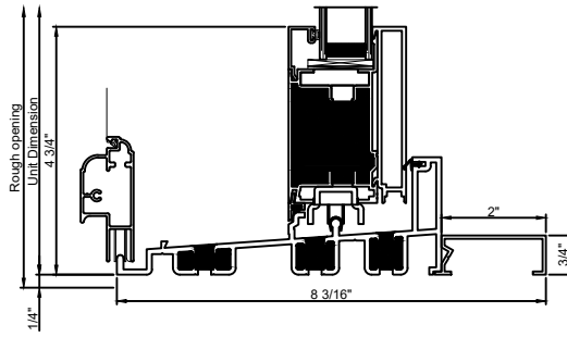
6 9/16" Std. Sill
