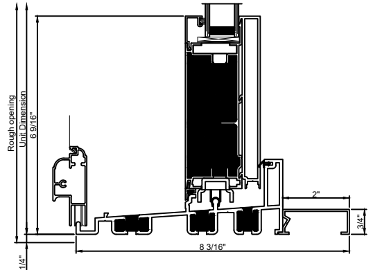
6 9/16" Std. Sill
